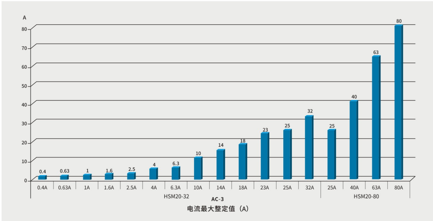
HSM20系列电动机保护断路器整定电流
