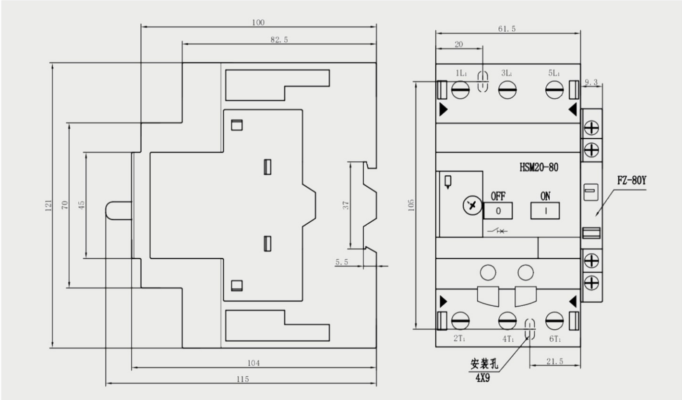
HSM20-80断路器及其附件安装尺寸外型图
