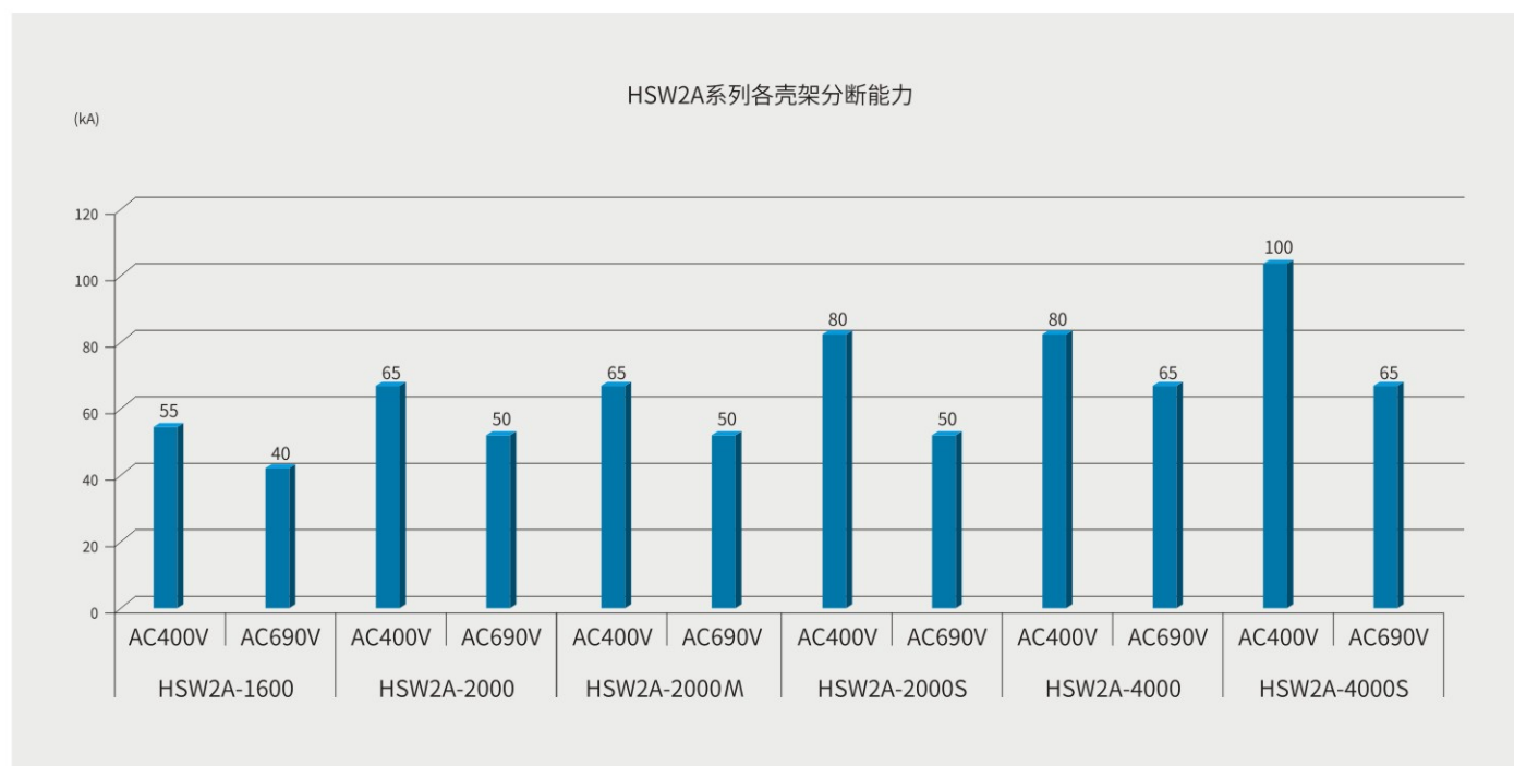
HSW2A系列各壳架分断能力
