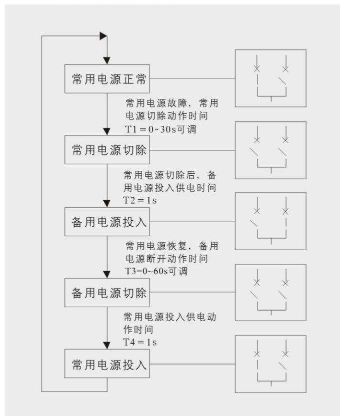
电网-电网型自投自复功能逻辑图
