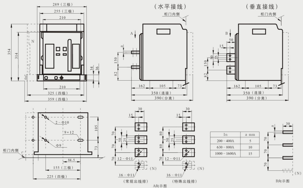
图9抽屉式断路器安装尺寸及外形尺寸 (HSW2A-1600、1600/4)
