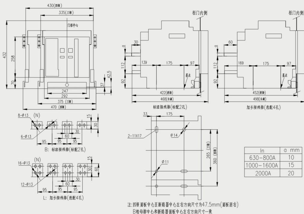
图11抽屉式断路器安装尺寸及外形尺寸 (HSW2A-2000、2000/4)
