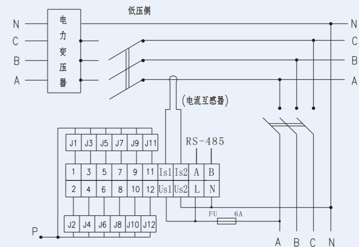
图三 42 方形控制器接线图 (AC220V 采样)
