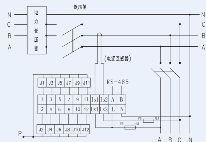
图四 42 方形控制器接线图 (AC380V 采样)
